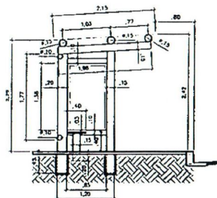
ELEVAÇÃO LATERAL ESCALA 1/50
