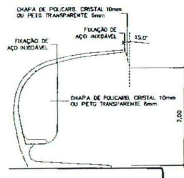
DET. FECHAMENTO LATERAL ESCALA 1/50
