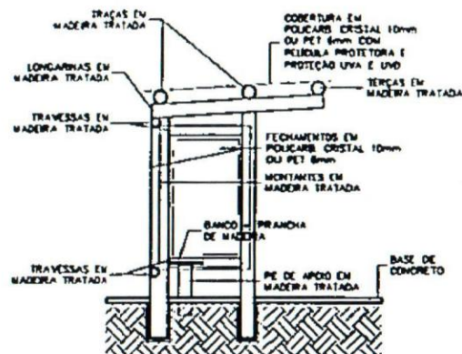
ELEVAÇÃO LATERAL ESCALA 1/50
