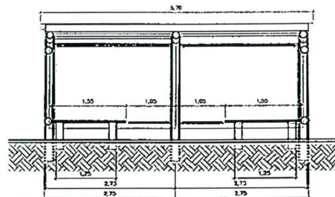
ELEVAÇÃO FRONTAL ESCALA 1/50
