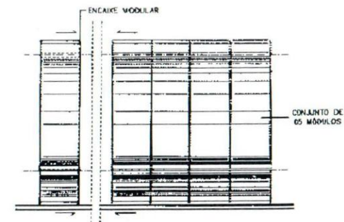
DET. JUNÇÃO DAS PEÇAS ESCALA 1/50
