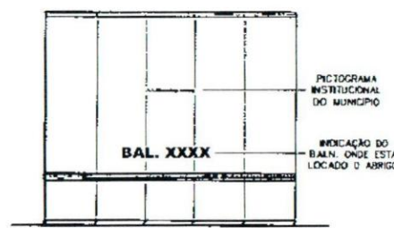
ELEVAÇÃO FRONTAL ESCALA 1/50
