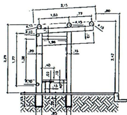
ELEVAÇÃO LATERAL ESCALA 1/50
