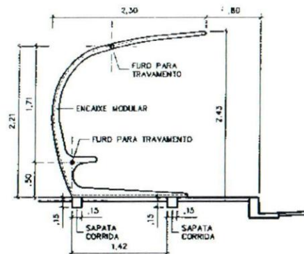
ELEVAÇÃO LATERAL ESCALA 1/50
