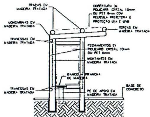
ELEVAÇÃO LATERAL ESCALA 1/50
