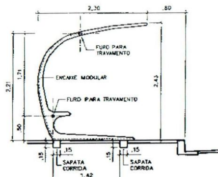
ELEVAÇÃO LATERAL ESCALA 1/50
