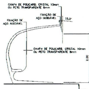
DET. FECHAMENTO LATERAL ESCALA 1/50
