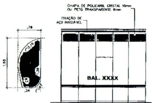
DET. FECHAMENTO FRONTAL ESCALA 1/50
